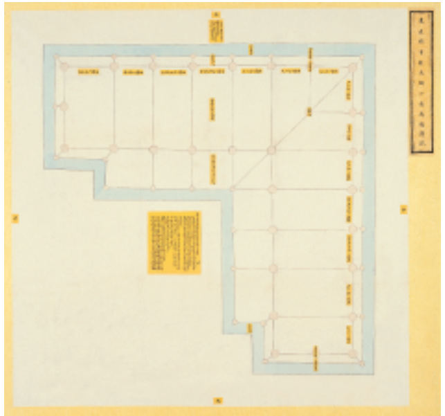
東直門重簷角樓一座底盤圖說（二） 紙本設色，原尺寸縱六九公分、橫六八·五公分。 圖上貼有黃籤，說明東直門建制。
