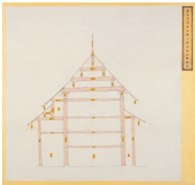
東直門重簷角樓一座大山木樣（三） 紙本設色，原尺寸縱六八·三公分、橫六八·三公分
