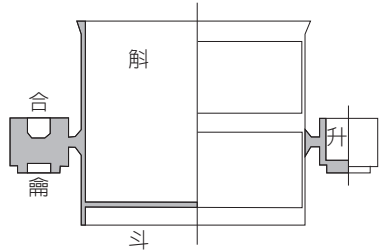
嘉量剖面示意圖
